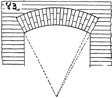
४३. Gauged arch : घडीव विटांची
